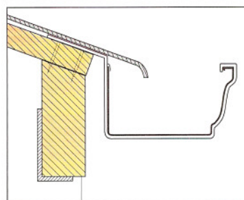
Buitenbeugels
