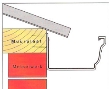
Gemonteerd aan de muurplaat met metselwerk.
