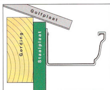
Aluminium dakgoot bevestigd aan de geprofileerde staalplaat.
